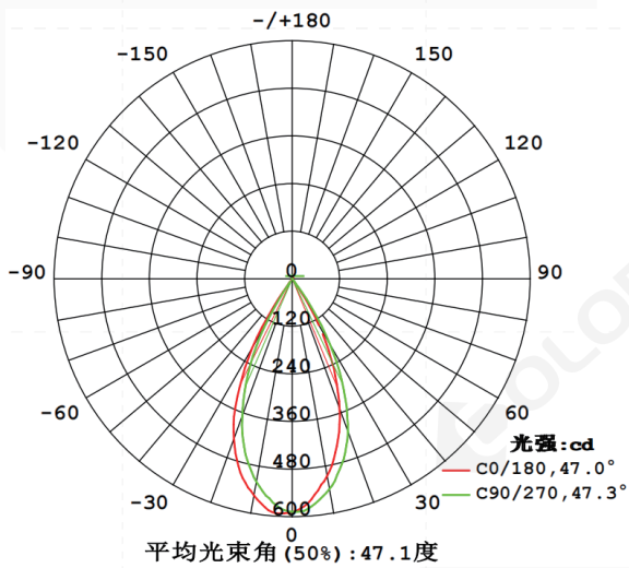
配光曲线图
