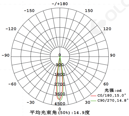
配光曲线图
