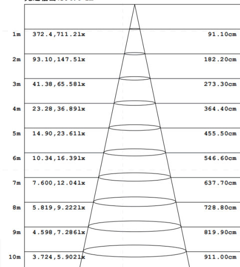
平均有效照度图
